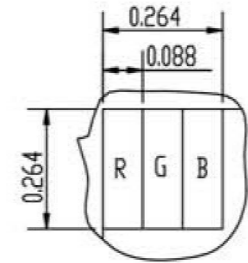
Detail A 60:1
