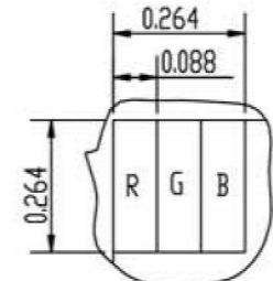
Detail A 60:1
